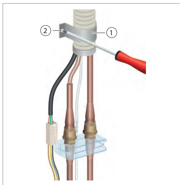
Abb. 13: Zugentlastung entfernen
