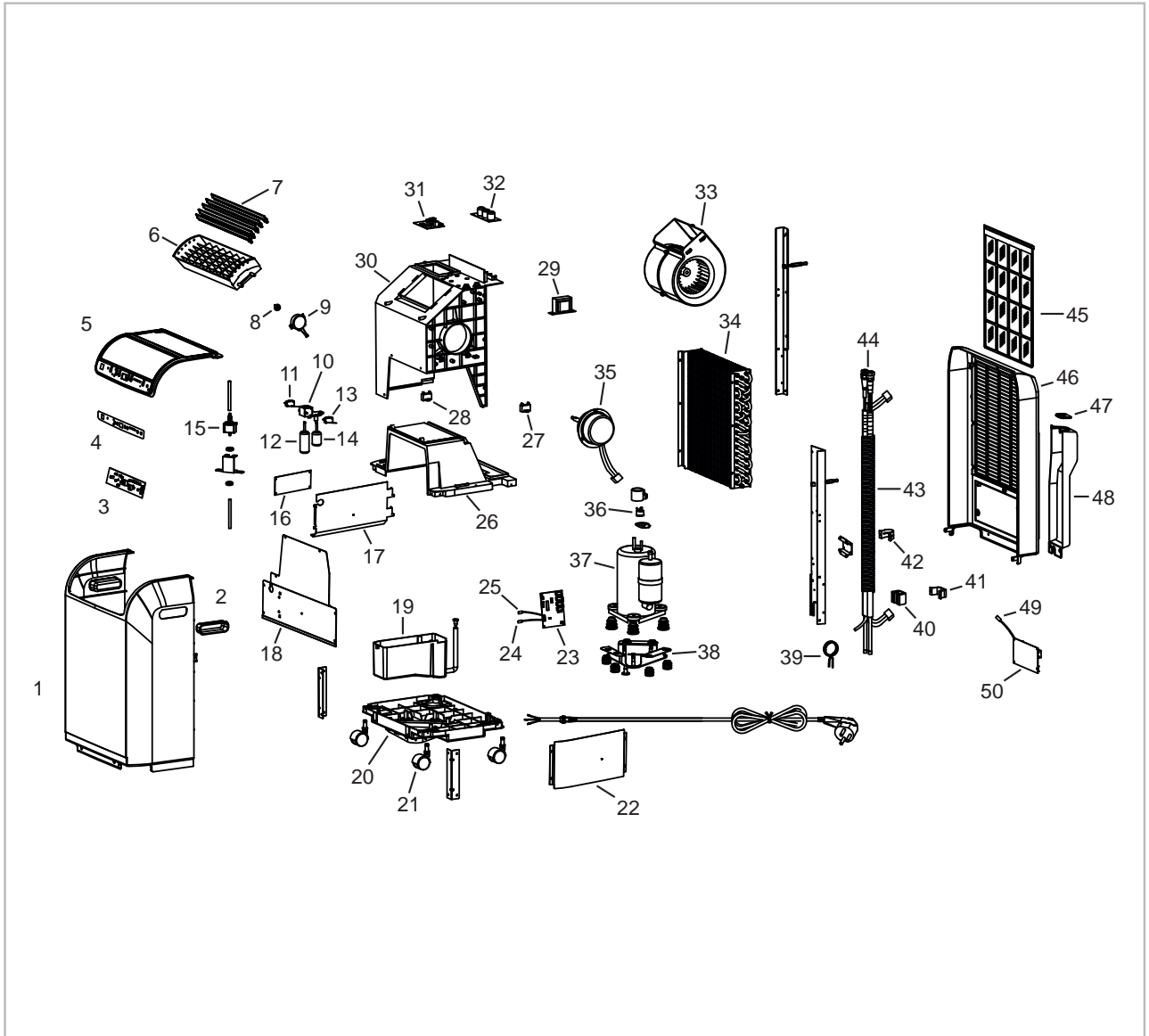
Abb. 21: Explosionszeichnung Innengerät
