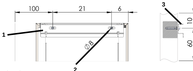
Afb 5: Overzicht wandmontage
