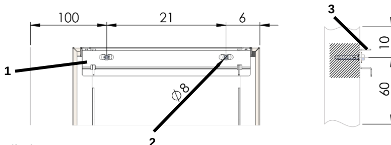
Fig 5: Översikt över väggfäste
