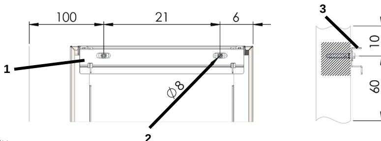
Fig 5: Oversikt veggfeste
