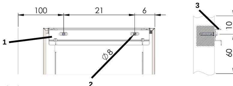
Fig 5: Übersicht Wandbefestigung
