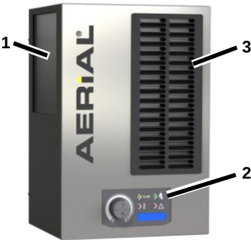
Fig. 1: Vista delantera
