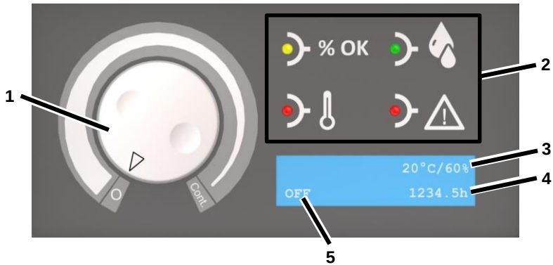
Fig. 4: Übersicht Bedienfeld
