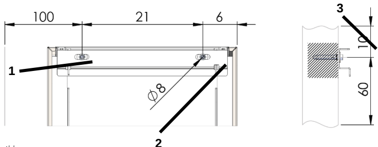
Fig. 5: Panoramica del fissaggio alla parete
