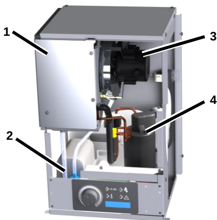
Fig. 3: Innenansicht
