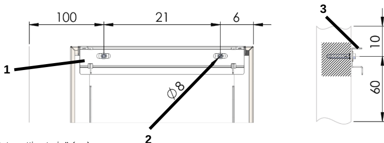
Kuva 5: Seinäkiinnityksen yleiskuva
