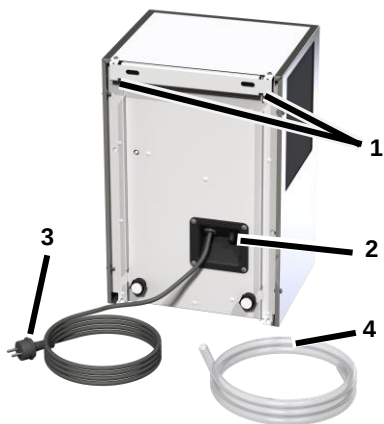
Rys. 2: Widok z tyłu
