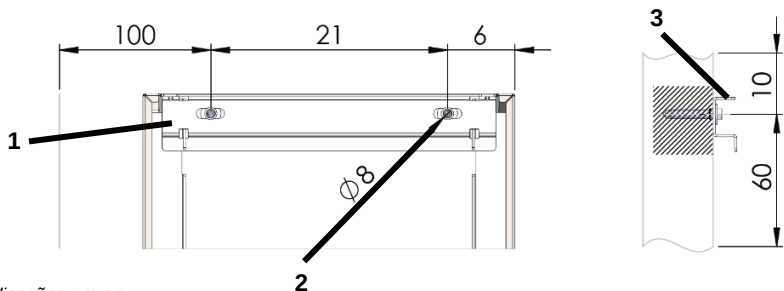
Fig 5: Vista geral da fixação de parede
