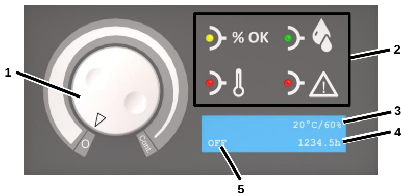
Fig. 4: Oversigt over betjeningspanel
